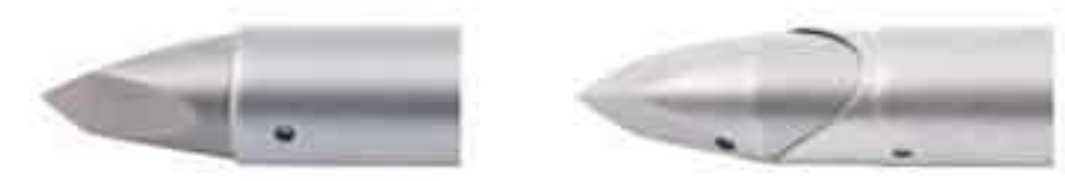
磁片式 Magnel E2016.12 Φ5.5mm E2016.13 Φ10.5mm E2016.14 Φ11mm E2016.15 Φ6mm E2016.16 Φ12mm E2016.19 Φ5.5mm 配 Stryker
