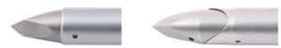
球阀式 Ball valve E2016.41 Φ5.5mm E2016.42 Φ6mm E2016.43 Φ10.5mm E2016.44 Φ11mm
